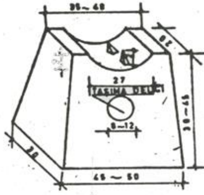
A-KÜÇÜK TİP BETON AYAK
