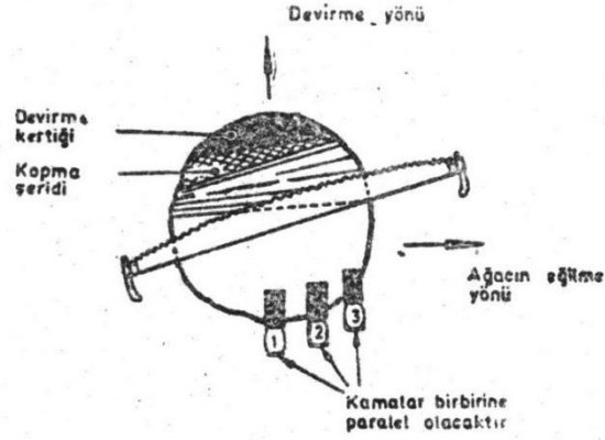
ŞEKİL-16 Devirme yönüne göre, yana eğik ağacın devirme kesişinin ağacın enine kesiti üzerindeki görünüşü.
