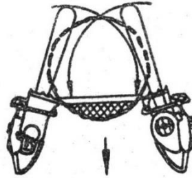
ŞEKİL-22 Dip çapı, motorlu testere levha uzunluğunun birbuçuk katına kadar olan normal duruşlu ağaçta devirme kesişinin yapılması.
