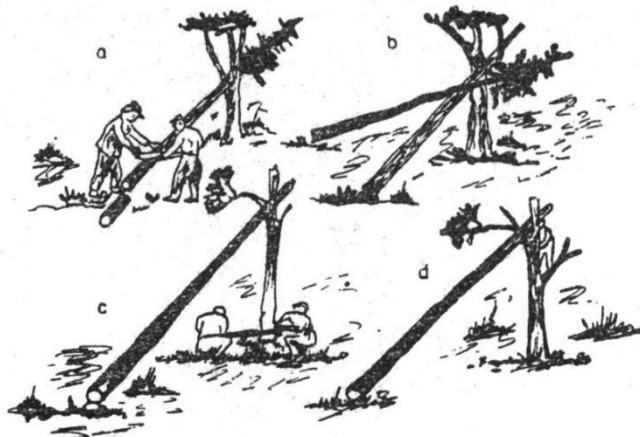
ŞEKİL-29 Devrilmesi sırasında çevredeki herhangi bir yere dayanan ağacın düşürülmesinde baş vurulması tehlikeli ve sakıncalı kurallardır.
