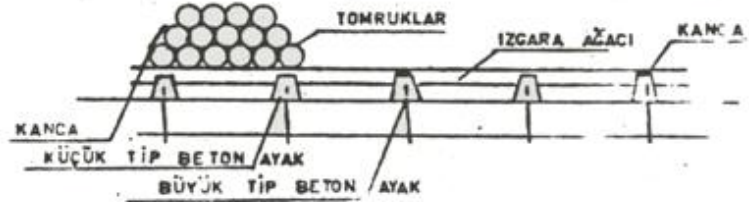
C-BETON AYAKLI DİREK IZGARALARIN YANDAN GÖRÜŞÜ VE KANCA DEMİRİ İLE BAĞLANTISI
