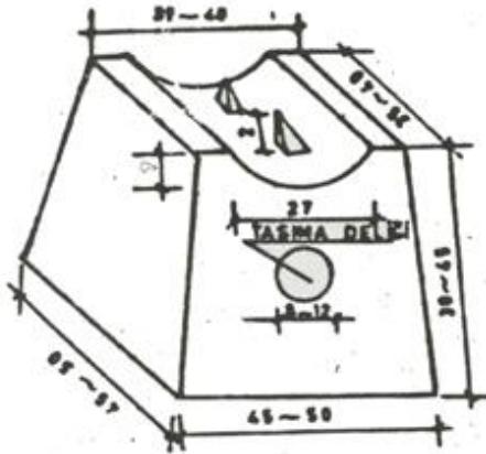
B-BÜYÜK TİP BETON AYAK
