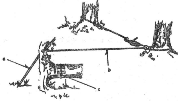
ŞEKİL-30 Rüzgâr ve kar devriklerinin topraklı kök kısmının geriye kapaklanmaması için: a = Arkadan desteklenmesi, b = Çekme gereciyle gergin olarak dikili bir ağaca bağlanması, c = Kesme sırasında gövdenin yarılmamasının istenmesi halinde gövde presliyle sıkılması.
