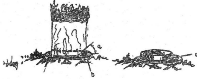
ŞEKİL-15 a = Devirme kertiği ağzı. b = Devirme kertiği tabanı. c = Devirme kertiği iç kenarı.
