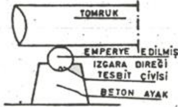
A-BETON AYAKLI DİREK IZGARALARIN ÖNDEN GÖRÜLEN DİK KESİTİ
