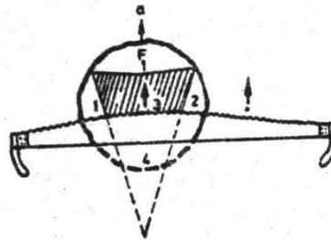
ŞEKİL-17 Devirme yönüne doğru eğik ağaçlarda devirme kesişinin enine kesit üzerinde görünüşü.
