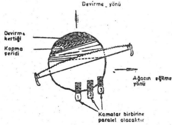
ŞEKİL-16 Devirme yönüne göre, yana eğik ağacın devirme kesişinin ağacın enine kesiti üzerinde görünüşü.
