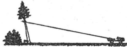
ŞEKİL - 19 Davirme yönünün aksi tarafına eğik ağacın yalnız kamalar yardımıyla kesilmesi.
