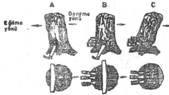
ŞEKİL - 19 Davirme yönünün aksi tarafına eğik ağacın yalnız kamalar yardımıyla kesilmesi.
